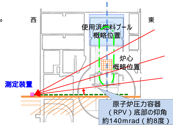
原子炉建屋を透過するミュオンの測定イメージ (東西断面図)
