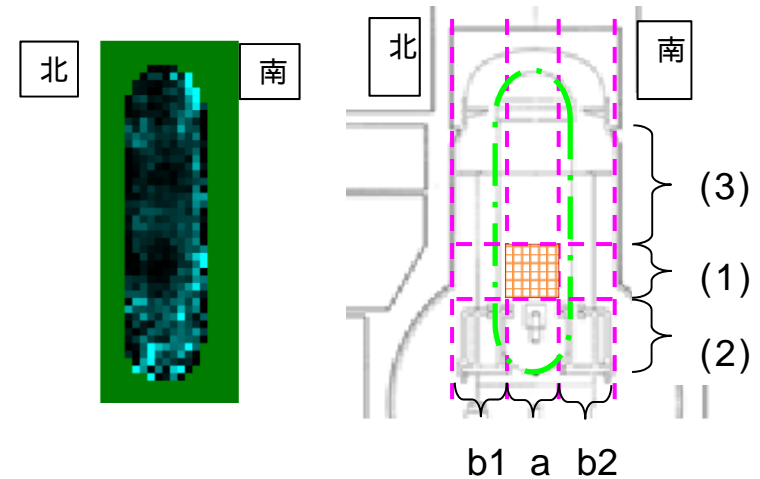
シミュレーションとの比較による物質量の評価
