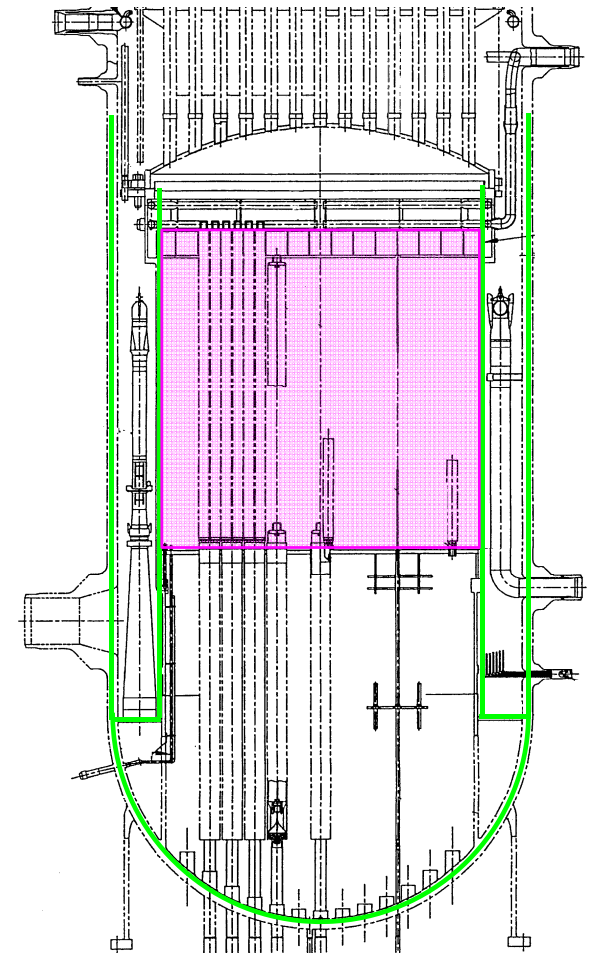
压力容器下部の構造
