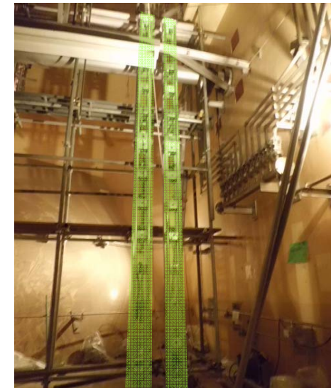
鋼製支柱設置状況(着色部が支柱) (32本中2本施工した状況)
