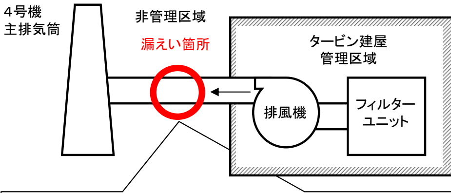
4号機主排気ダクト支持脚溶接部における 空気の漏えい箇所（平成23年6月7日確認）
